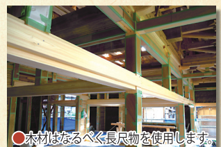
●貫甲造り
